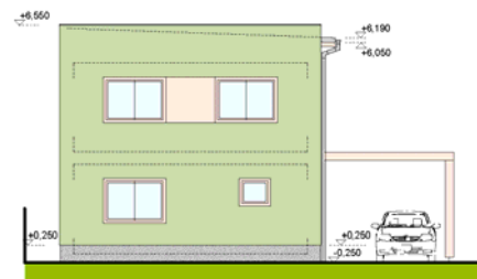
POHLED SEVEROVÝCHODNÍ
